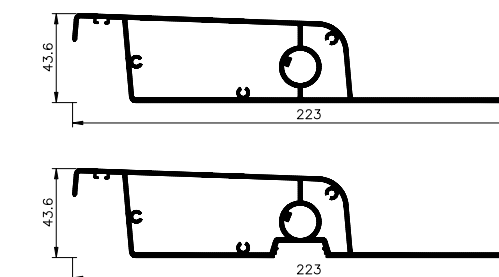
Daklamel met de afmetingen 44×223 mm
